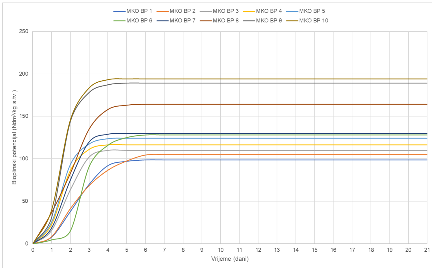
Slika 8. Bioplinski potencijal ispitanih uzoraka miješanog komunalnog otpada.
