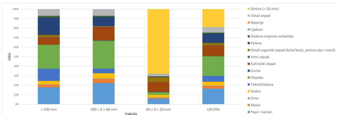
Slika 6. Morfološke sastavnice reprezentativnog uzorka miješanog komunalnog otpada po frakcijama.
