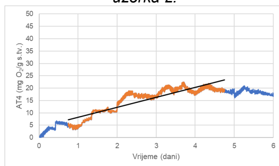
Slika 13. Respiracijska aktivnost AT_4 uzorka 4.
