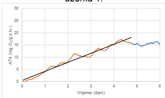
Slika 12. Respiracijska aktivnost AT_4 uzorka 3.
