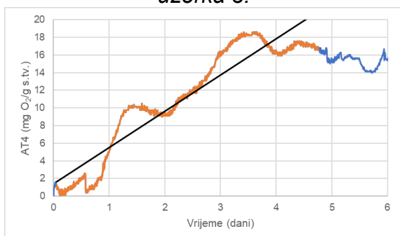
Slika 14. Respiracijska aktivnost AT_4 uzorka 5.
