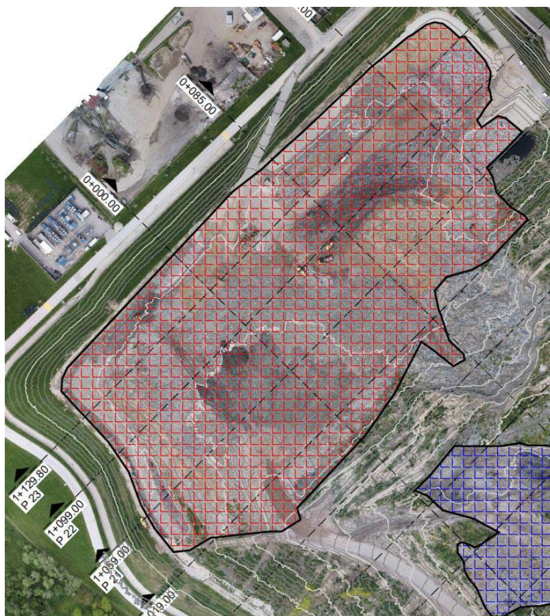
Slika 1. Područje na kojemu je proveden proračun volumena otpada ugrađenog na plohi 6/3.
