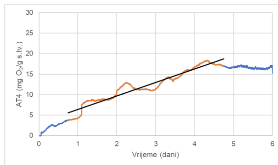
Slika 11. Respiracijska aktivnost AT_4 uzorka 2.
