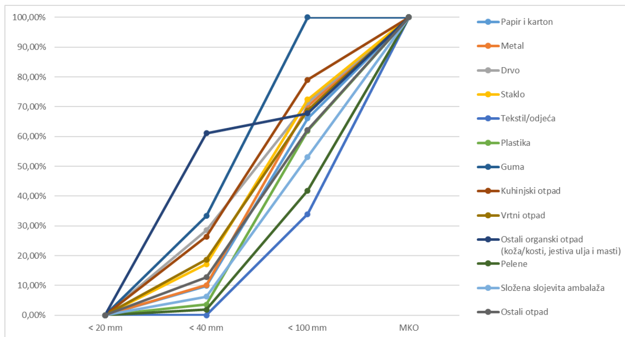
Slika 7. Maseni udjeli morfoloških sastavnica otpada prosijanih kroz sito po frakcijama otpada ( > 100 , 100 > x > 40 , 40 > x > 20 ) za reprezentativni uzorak miješanog komunalnog otpada.
