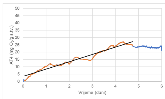
Slika 19. Respiracijska aktivnost AT_4 uzorka 10.
