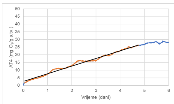
Slika 18. Respiracijska aktivnost AT_4 uzorka 9.
