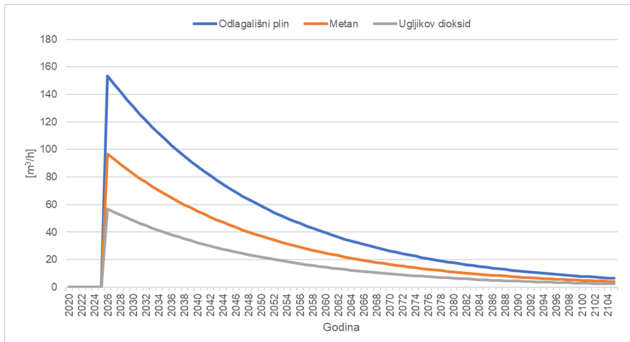
Slika 21. Proizvodnja odlagališnog plina iz otpada odloženog tijekom 2025. godine.
