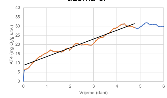
Slika 17. Respiracijska aktivnost AT_4 uzorka 8.
