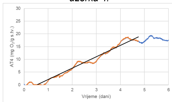
Slika 15. Respiracijska aktivnost AT_4 uzorka 6.
