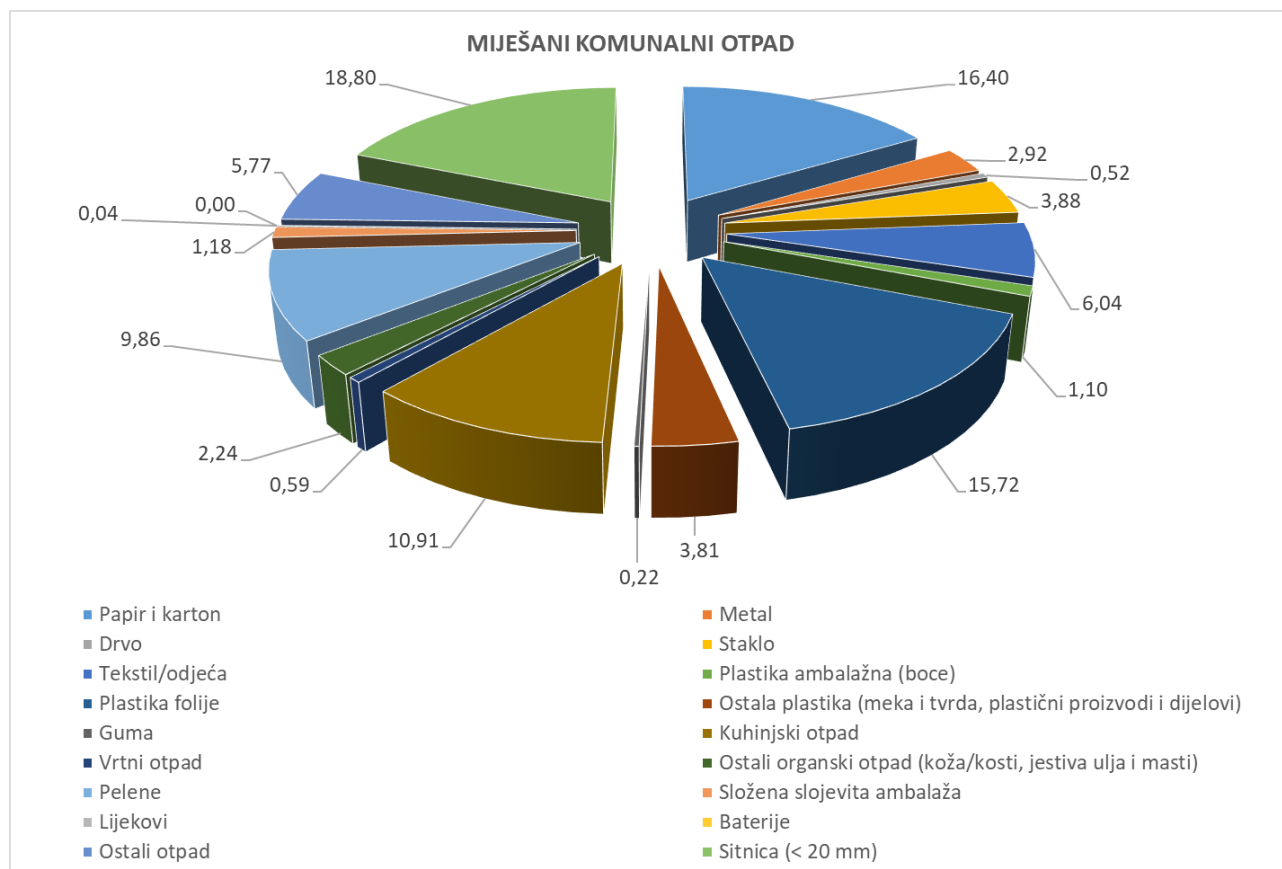
Slika 4. Morfološke sastavnice reprezentativnog uzorka miješanog komunalnog otpada – sekundarne sastavnice otpada.
