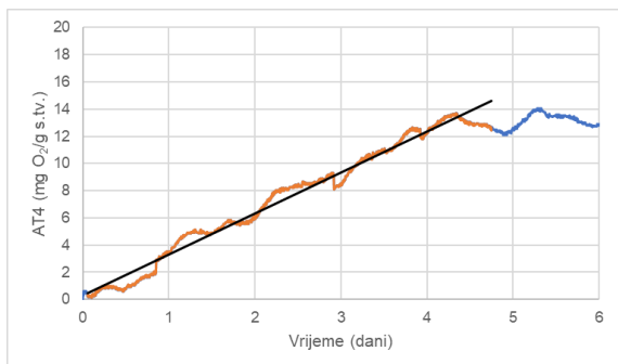
Slika 10. Respiracijska aktivnost AT_4 uzorka 1.
