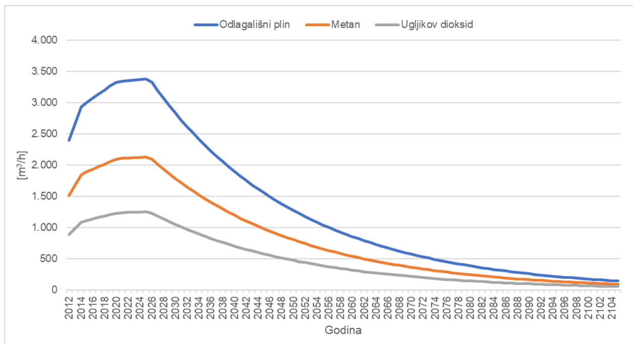
Slika 20. Proizvodnja odlagališnog plina iz odloženog otpada tijekom godina.
