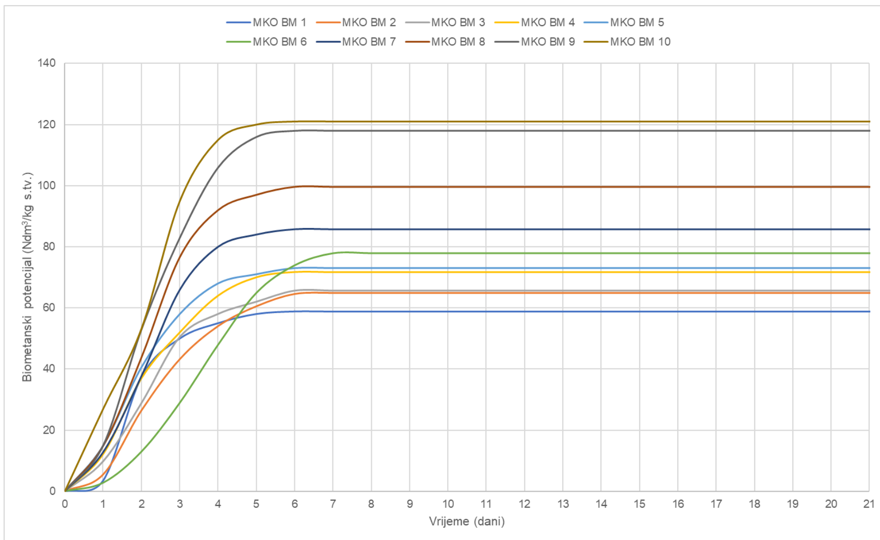
Slika 9. Biomatanski potencijal ispitanih uzoraka miješanog komunalnog otpada.
